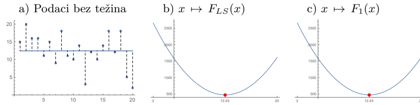
Slika 9.1: Najbolji LS-reprezentant i najbolji \ell_1 -reprezentant skupa podataka \mathcal{A} \subset \mathbb{R}
