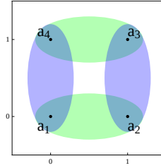
Slika 3.7: LS-optimalne particije
