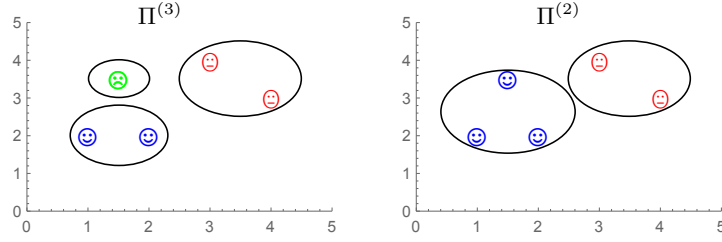
Slika 5.1: Particija \Pi^{(3)} je ugnježena u particiju \Pi^{(2)} ( \Pi^{(3)} \sqsubset \Pi^{(2)} )
