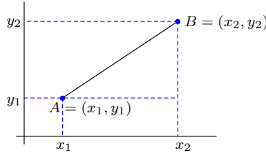
Slika 8.11: Udaljenost točaka A, B u ravni
