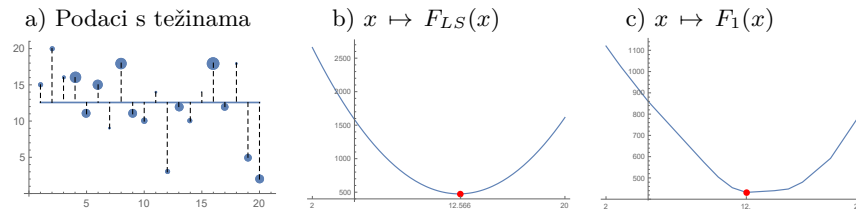
Slika 9.2: Najbolji težinski LS-reprezentant i najbolji težinski \ell_1 -reprezentant skupa podataka \mathcal{A} \subset \mathbb{R}
