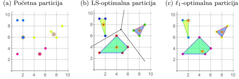
Slika 4.15: k -means iterativni proces
