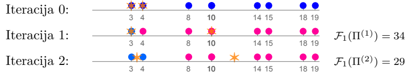
Slika 4.19: Traženje \ell_1 -optimalne 2-particije skupa \mathcal{A} = \{3, 4, 8, 10, 14, 15, 18, 19\}
