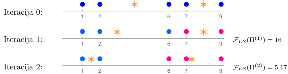
Slika 4.3: Traženje LS-optimalne 2-particije skupa \mathcal{A} = \{1, 2, 6, 7, 9\}
