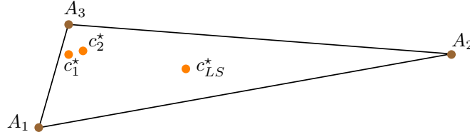
Slika 2.3: Fermat–Torricelli–Weberov problem ( c_2^* - geometrijski medijan, c_{LS}^* - centroid, c_1^* - medijan)
