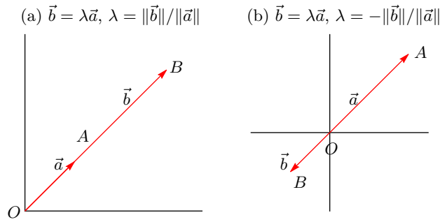
Slika 8.4: Kolinearni vektori
