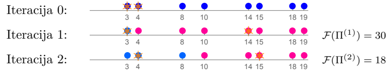
Slika 4.5: k -means algoritam uz primjenu \ell_1 -metričke funkcije
