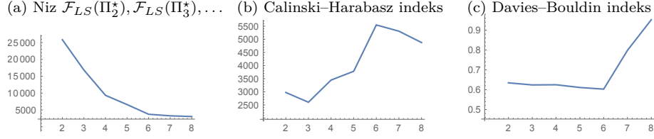
Slika 6.1: Izbor particije s najprikladnijim brojem klastera iz Primjera 3.2
