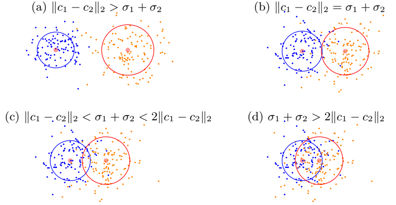
Slika 6.3: Međusobno različiti odnosi dva sferična skupa podataka
